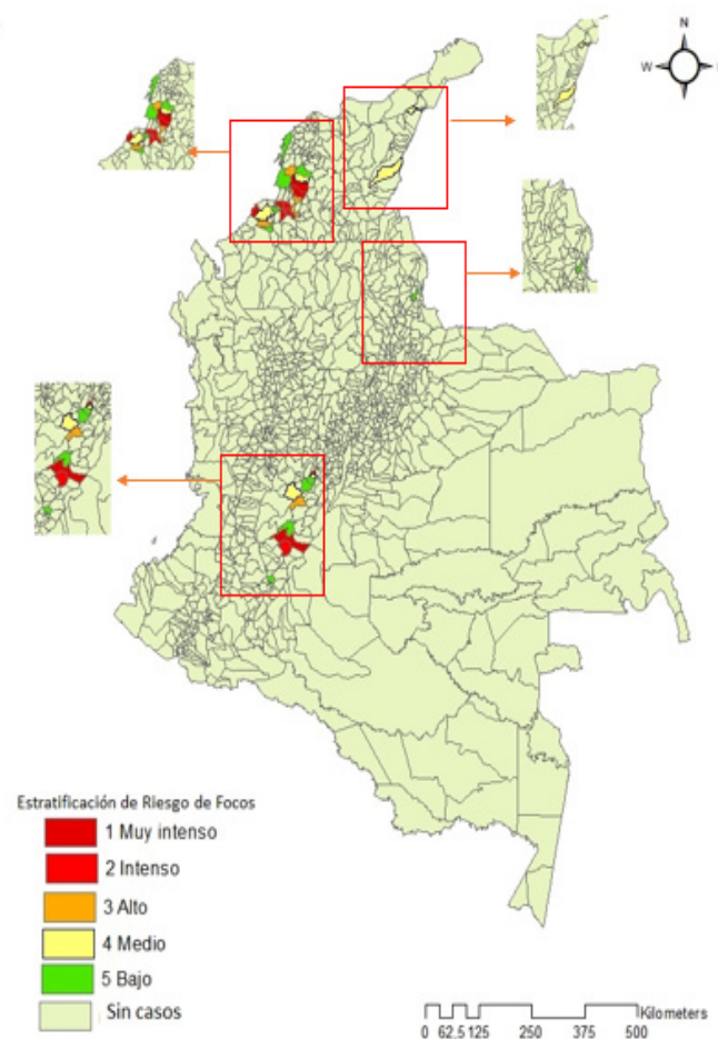
Mapa 1. Distribución geográfica de casos confirmados para L. visceral . Colombia, 2008-2018
